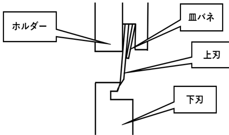
ゲーベル方式の刃組簡易図
