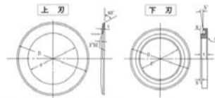
スリッターナイフ標準品 (ゲージベル型)
